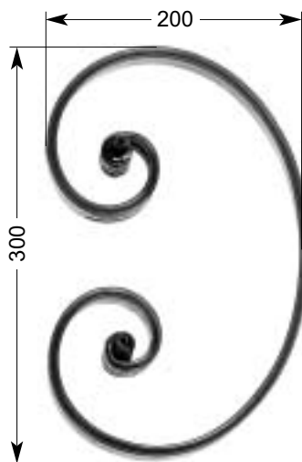
25 203 1,03 kg □ 16 x 8 mm
