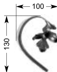
25 284 0,25 kg □ 16 x 8 mm
