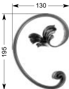
25 222 0,49 kg □ 16 x 8 mm
