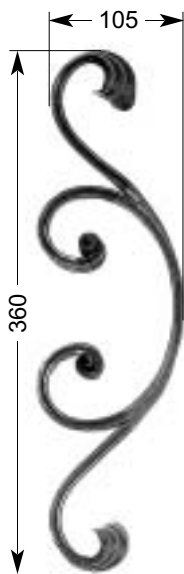
25 204 0,82 kg □ 16 x 8 mm
