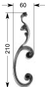
25 226 0,35 kg □ 16 x 8 mm
