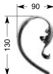
25 286 0,21 kg □ 16 x 8 mm
