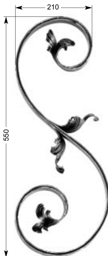
25 262 1,43 kg □ 16 x 8 mm
