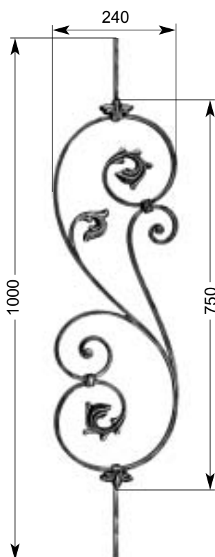
36 001 3,68 kg □ 16 x 8 mm
