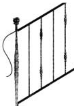
30 509 6,30 kg □ 20 x 20 mm
