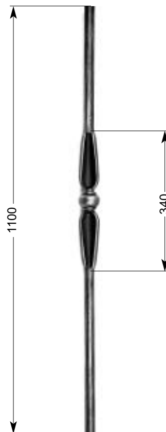
30 307 Anfangsstab mit Messingkugel Endpost, with brass ball Balustre de départ, boule en laiton 4,72 kg Ø 25 mm
