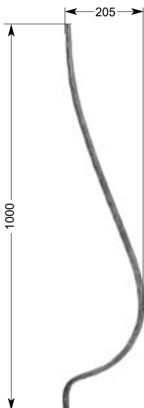
32 301 1,79 kg □ 13 x 13 mm
