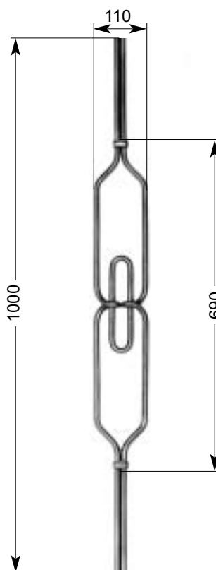
36 420 2,56 kg Ø 12 mm
