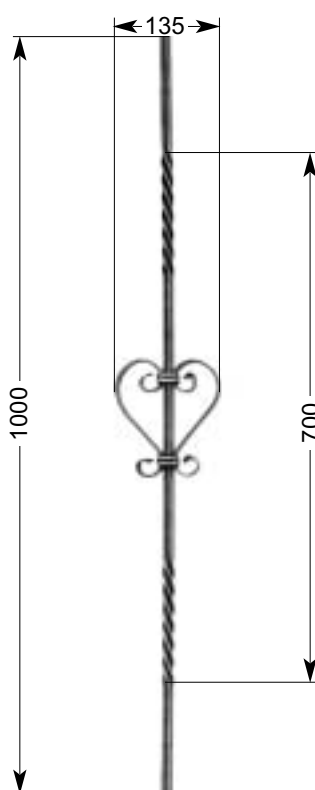
34 613 1,25 kg □ 12 x 12 mm
