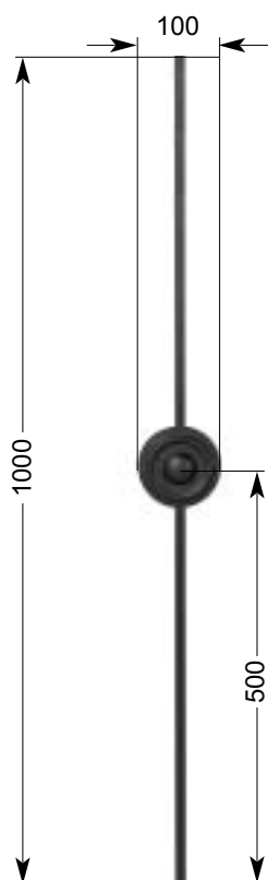
36 204 1,50 kg □ 12 x 12 mm
