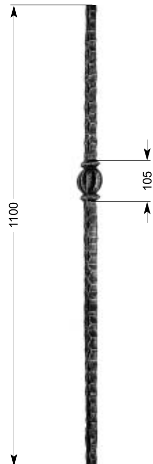
30 504 Anfangsstab Endpost Balustre de départ 5,10 kg □ 20 x 20 mm
