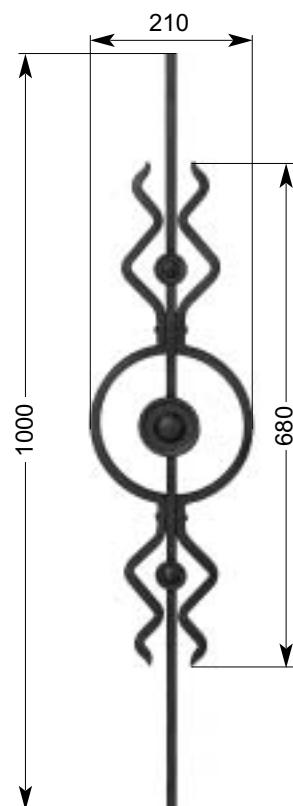
36 207 3,30 kg □ 12 x 12 mm
