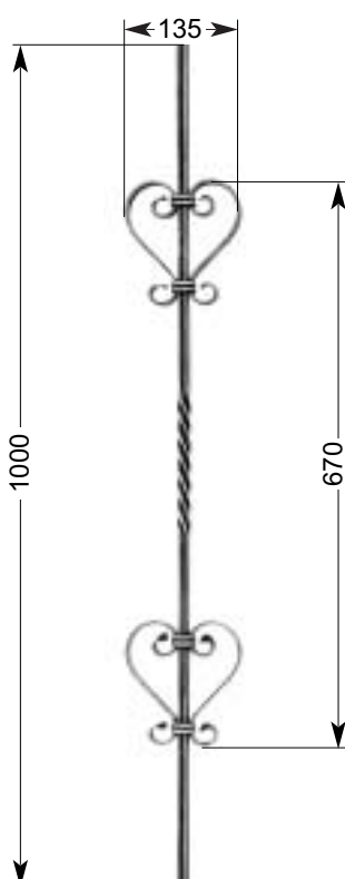
34 614 1,51 kg □ 12 x 12 mm
