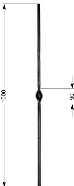
35 621 1,18 kg Ø 14 mm
