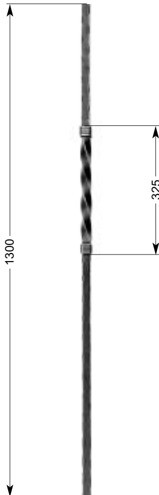
30 305 4,25 kg □ 20 x 20 mm
