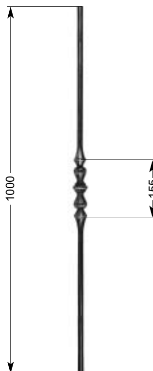
33 555* 1,85 kg Ø 14 mm
