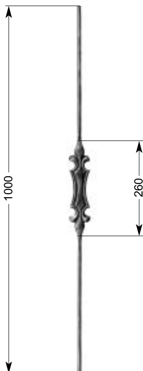
31 110 1,40 kg □ 16 x 8 mm
