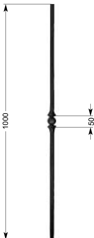
33 557* 1,55 kg □ 13 x 13 mm
