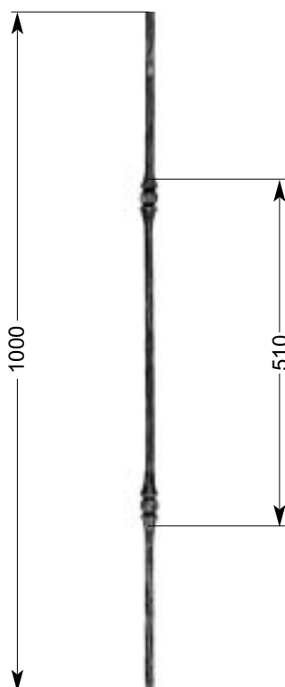
33 542 1,50 kg Ø 14 mm
