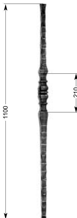
30 508 Anfangsstab Endpost Balustre de départ 6,13 kg □ 20 x 20 mm
