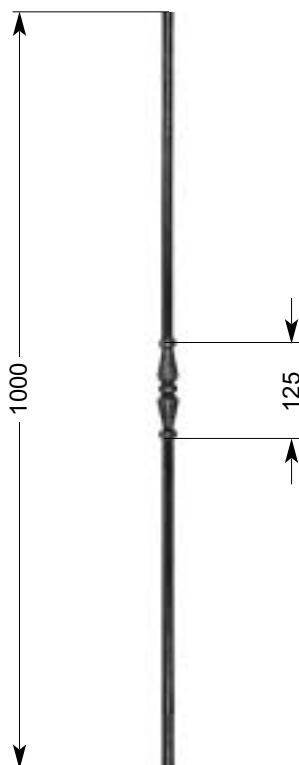
33 554* 1,20 kg Ø 12 mm
