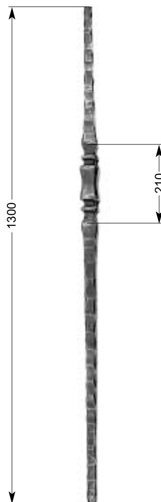
30 505 Anfangsstab Endpost Balustre de départ 7,20 kg □ 20 x 20 mm
