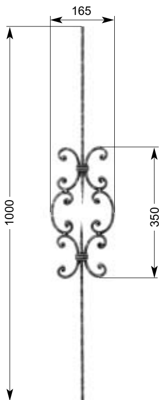
35 401 2,24 kg □ 16 x 8 mm
