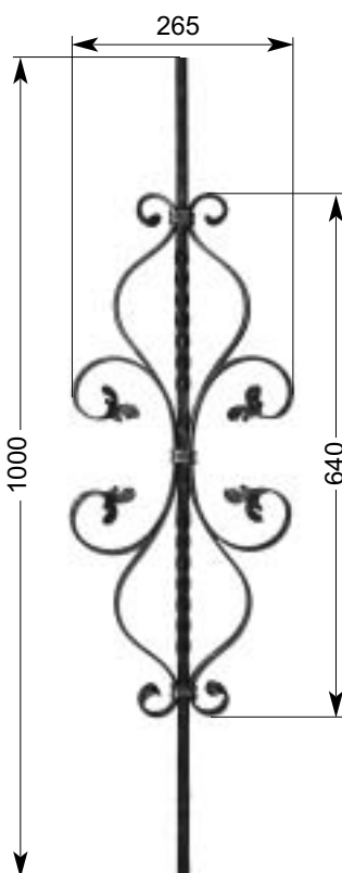
35 003 2,29 kg □ 12 x 12 mm
