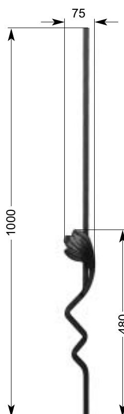
36 203 1,30 kg □ 12 x 12 mm
