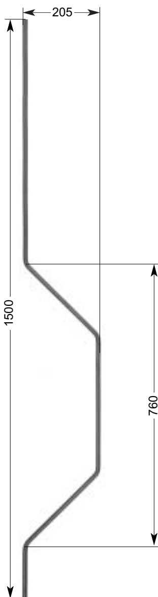
32 101 1,45 kg Ø 12 mm
