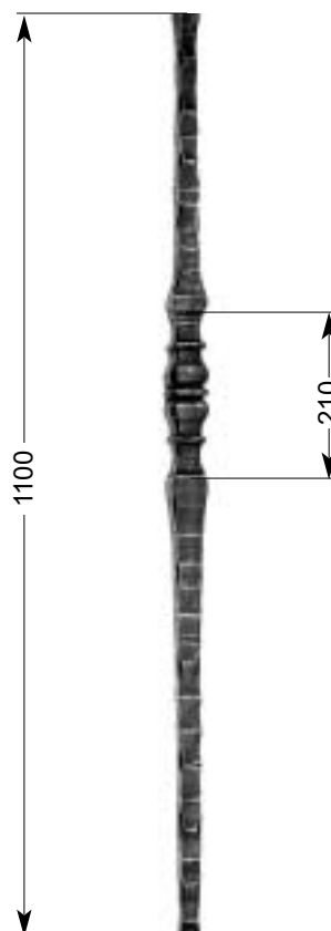
17 745* Handlaufverzierung Handrail ornament Ornement de main-courante 3,30 kg Ø 90 mm
