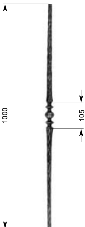
33 543 2,03 kg Ø 13 mm
