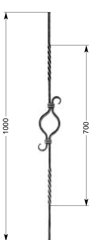
34 618 1,38 kg □ 12 x 12 mm
