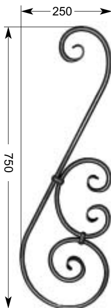
17 756 2,97 kg Ø 14 mm
