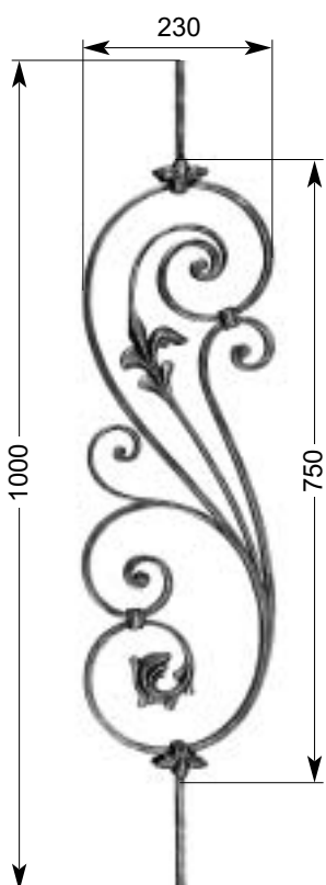
36 002 4,21 kg □ 16 x 8 mm
