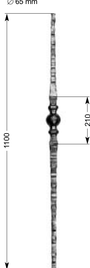
30 507 Anfangsstab Endpost Balustre de départ 8,10 kg □ 20 x 20 mm
