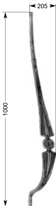
32 302 1,85 kg □ 13 x 10 mm
