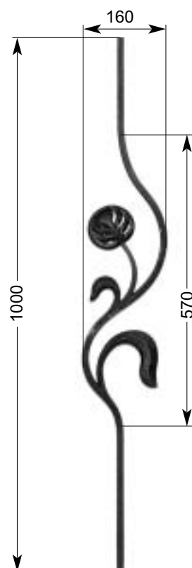
36 227 1,80 kg □ 12 x 12 mm
