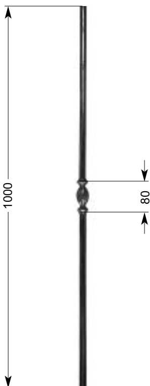
33 553* 1,10 kg Ø 12 mm
