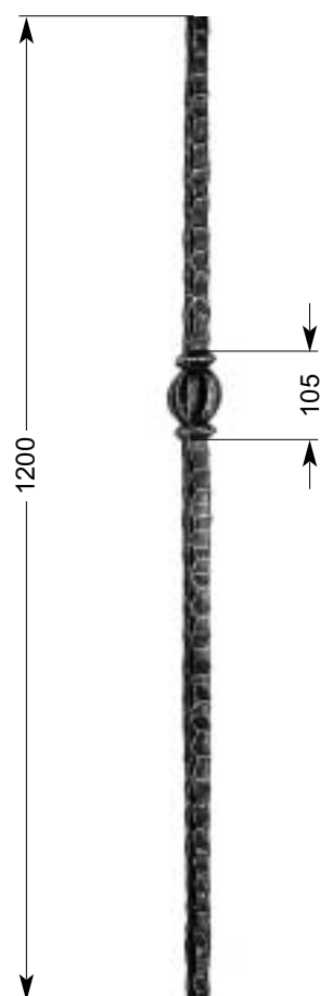
30 504 Anfangsstab Endpost Balustre de départ 5,10 kg □ 20 x 20 mm
