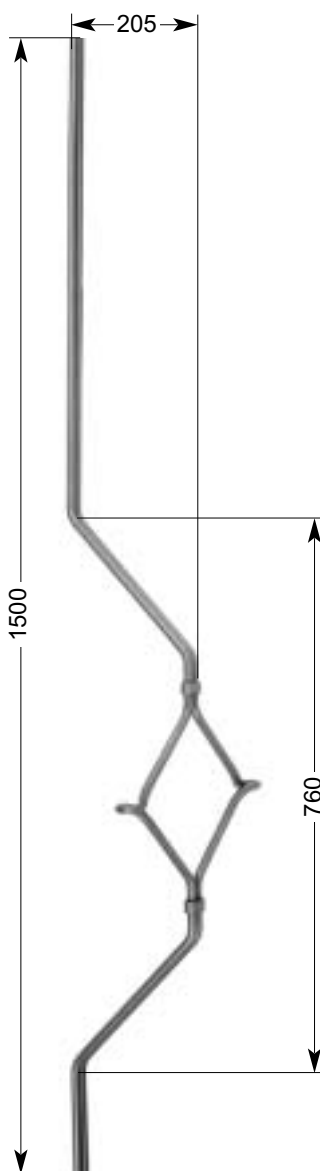
32 102 3,25 kg Ø 12 mm
