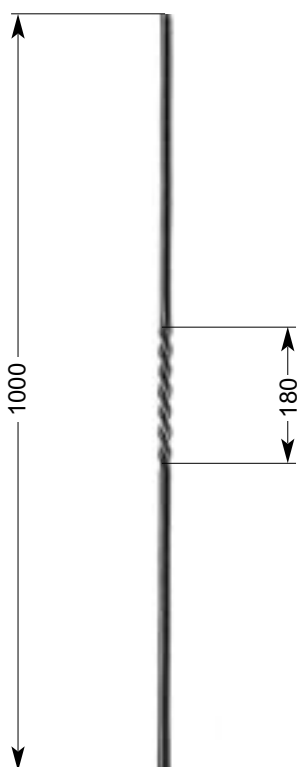
34 613 1,30 kg □ 14 x 14 mm
