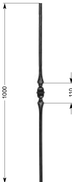
33 556* 1,75 kg Ø 14 mm
