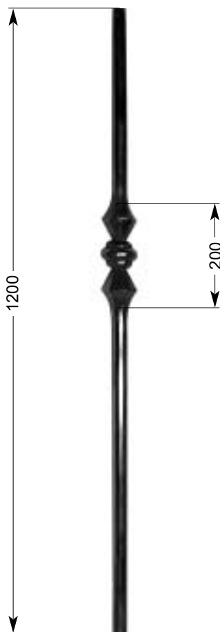
30 516* Anfangsstab Endpost Balustre de départ 7,20 kg Ø 25 mm
