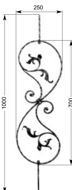
35 408 2,57 kg □ 16 x 8 mm
