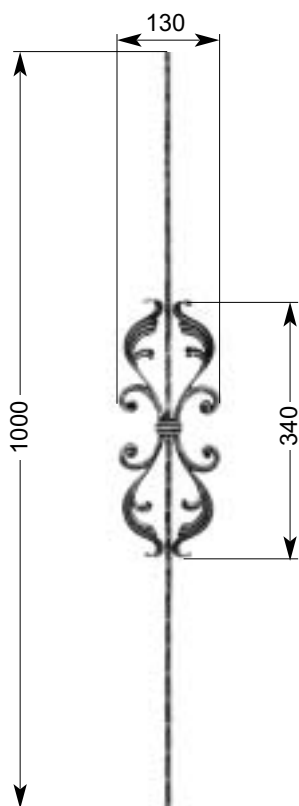
35 406 1,88 kg □ 16 x 8 mm
